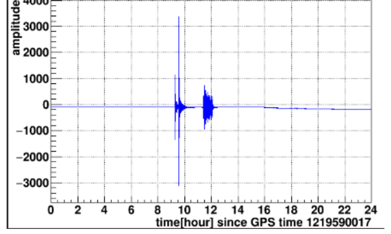
K1:VIS-ITMX_IP_DAMP_Y_IN1_DQ
