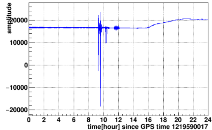
K1:VIS-ITMX_BF_DAMP_Y_IN1_DQ
