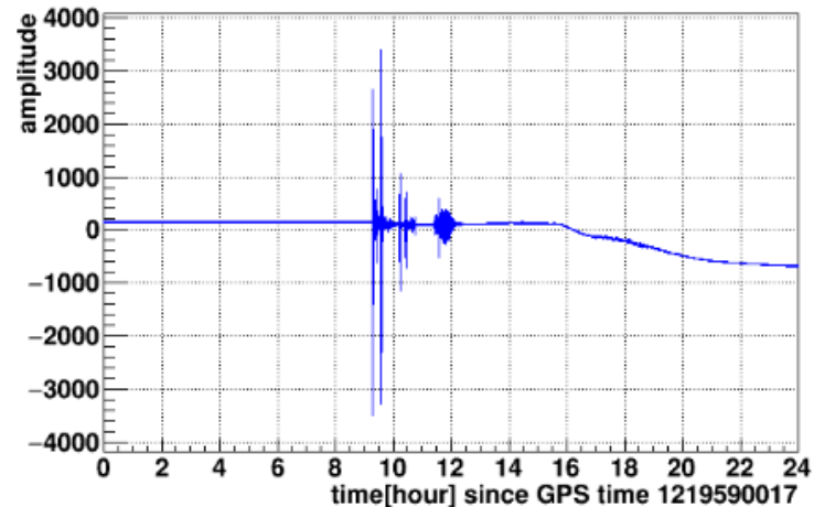
K1:VIS-ITMX_BF_DAMP_T_IN1_DQ
